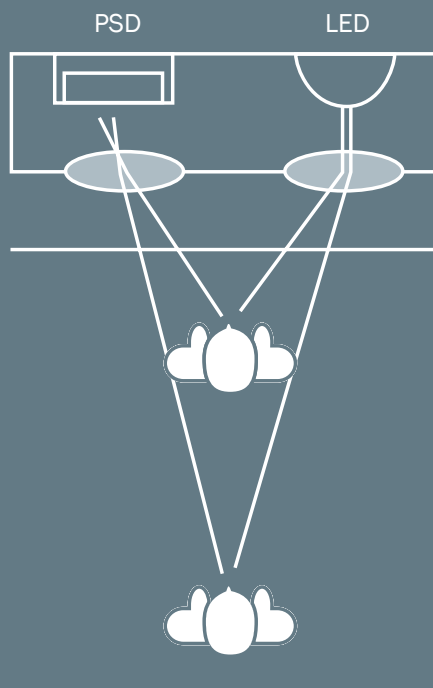
Tecnologia PSD di TECE con dissolvenza dello sfondo; funzionamento
